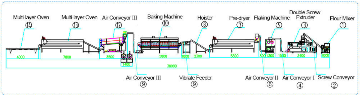
diagrama de flujo del proceso de fabricación de hojuelas de maíz
